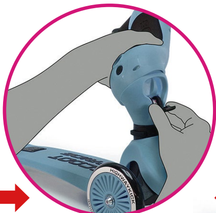
【スタンドモード】 高さ調整3段階 (ハンドル高さ 57～64cm)
